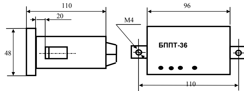
Рис.1 Щитовой монтаж
