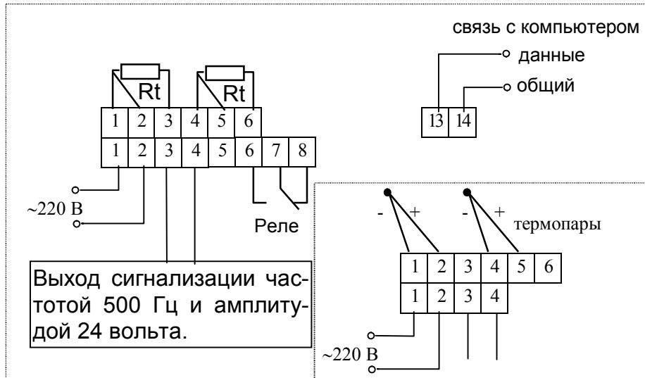
Рис.2а Исполнение с клеммными колодками
