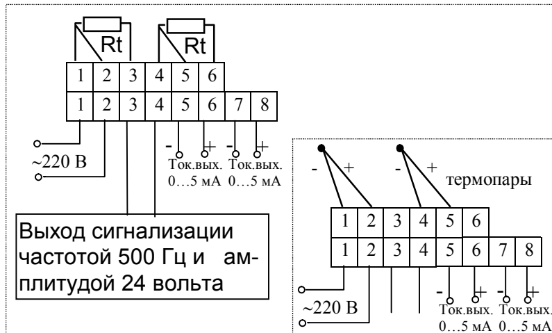
Рис.2б Исполнение с клеммными колодками и токовым выходом
