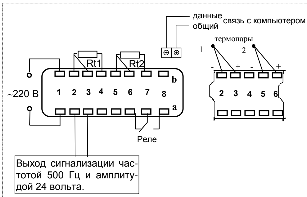
Рис.2в Исполнение с разъемом РП14-16
