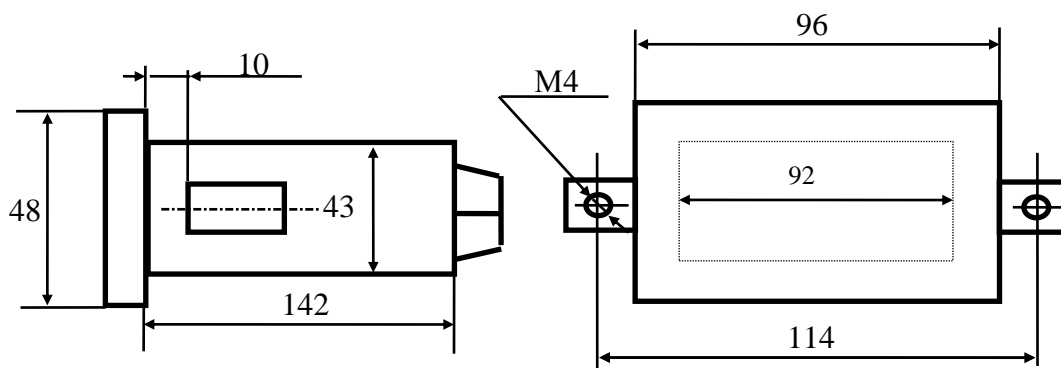
Рис. 4а Габаритные размеры, корпус 48x96x155 мм.
