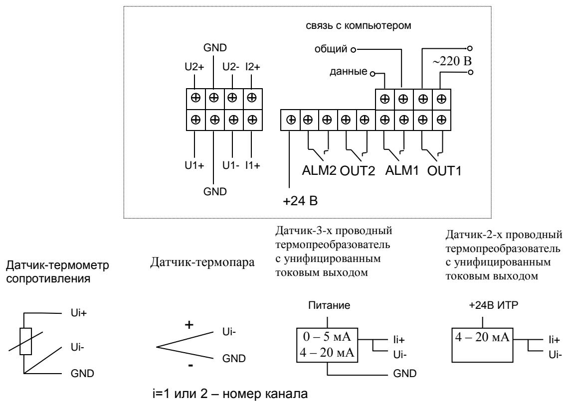
Рис. 3а Схема подключения с клеммными колодками (корпус 48x96x155мм).
