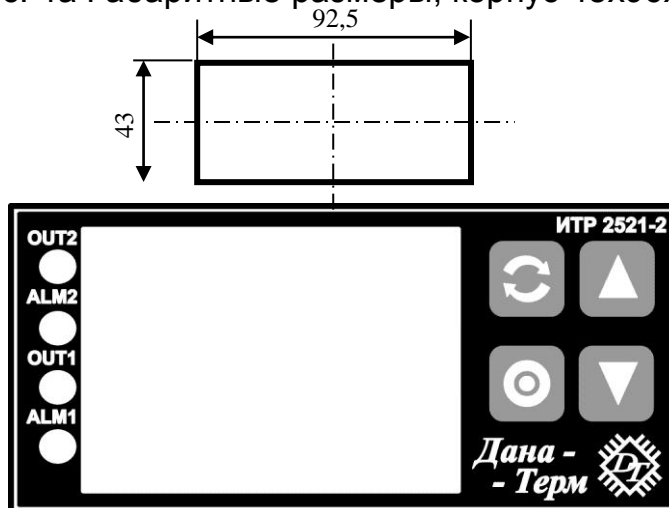
Рис. 4а Габаритные размеры, корпус 48x96x155 мм.
