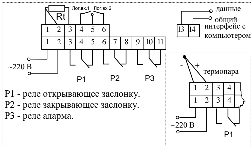
Рис. 2-1 Исполнение с клеммными колодками
