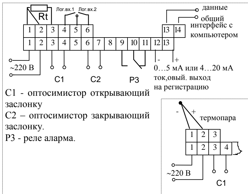
Рис. 2-2 Исполнение с клеммными колодками (с оптосимисторами) с выходом на регистрацию
