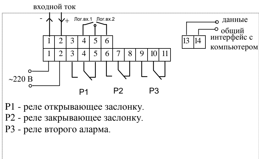
Рис. 2-3 Исполнение с клеммными колодками с токовым входом
