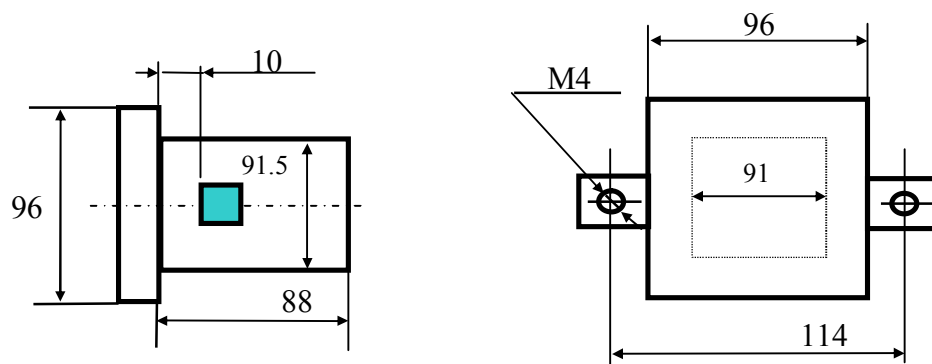
Рис. 4в Габаритные размеры, корпус 96x96x96 мм.
