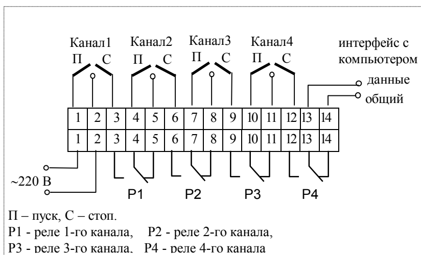
Рис.3 Исполнение с клемными колодками
